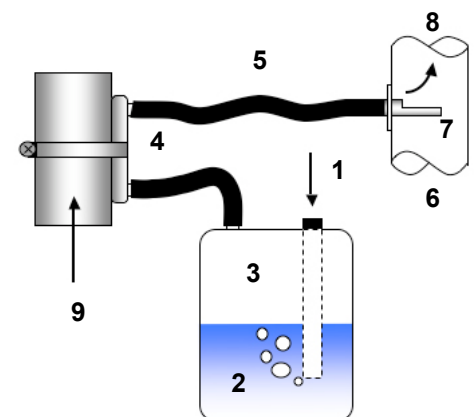
Réacteur Retrokit® Nano-Pro, montage extérieur au tube d'échappement
